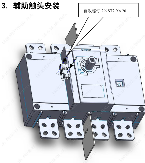
辅助触头安装 (一个)
