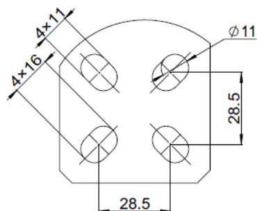
接线排尺寸
