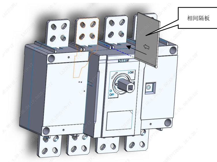
基本型产品相间隔板安装
