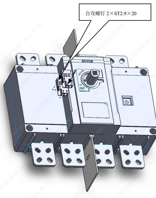
辅助触头安装 (二个)
